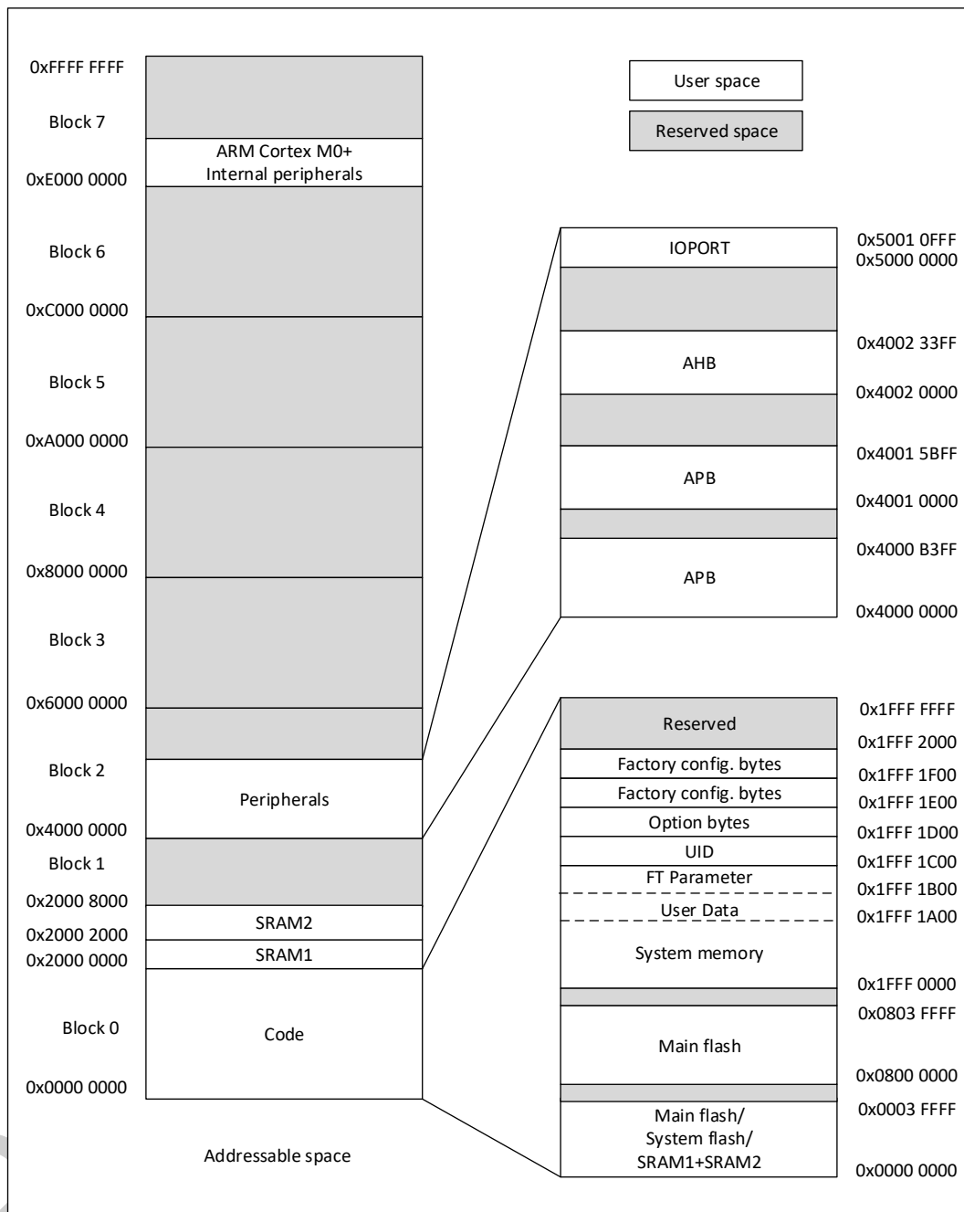
图 4-1 存储器映射
