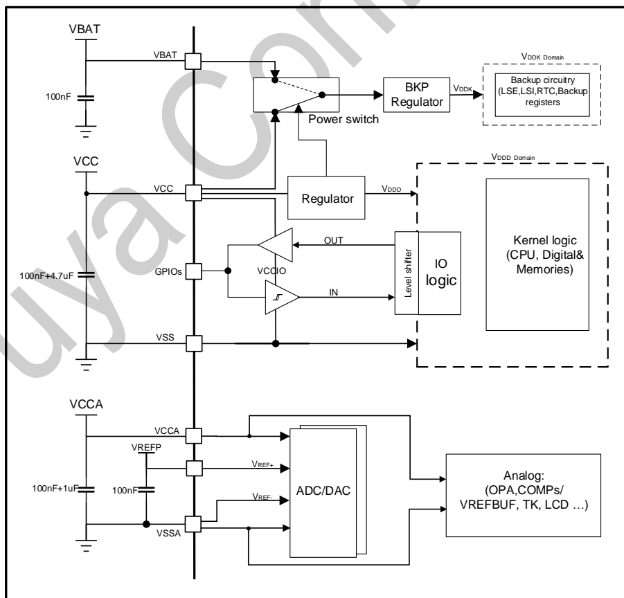
图 5-1 供电方案图
